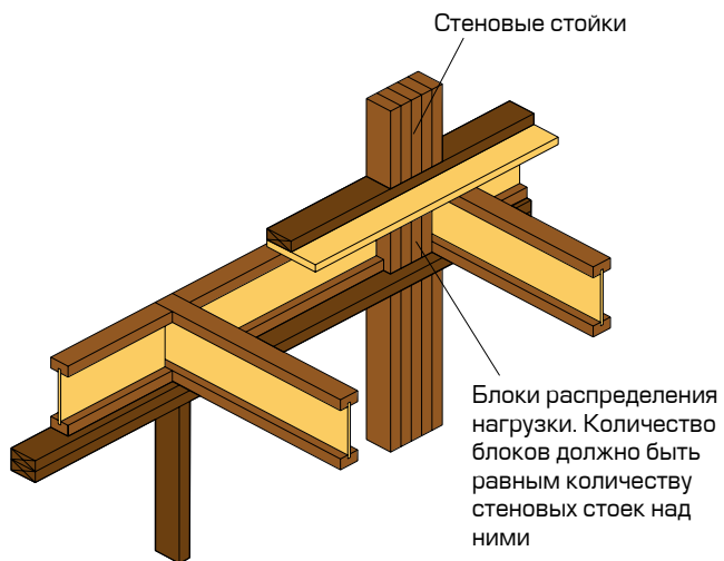
15 Устройство консоли (серии БДКУ/БДКШ)
