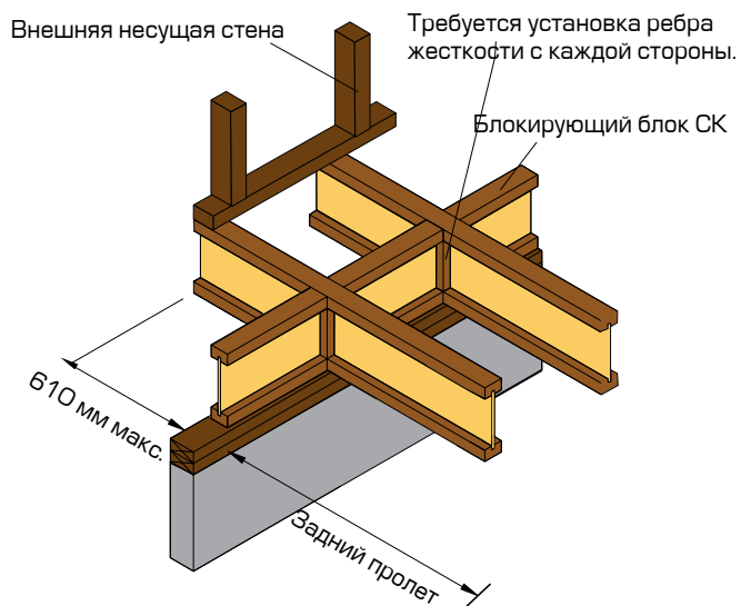
15 Устройство консоли (серии БДКУ/БДКШ)
